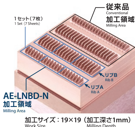
加工形状 Work Shape
